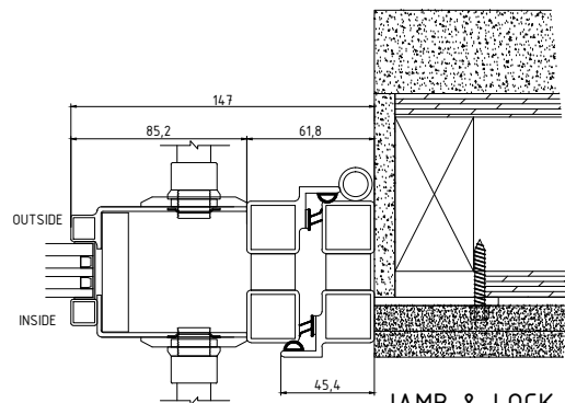
JAMB & LOCK
