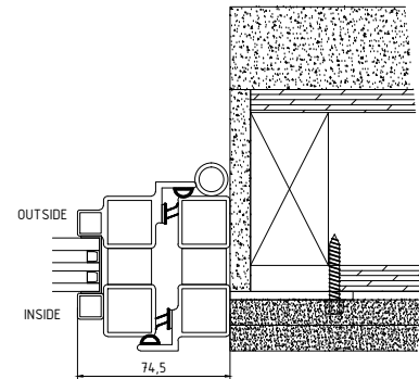
JAMB & STILE
