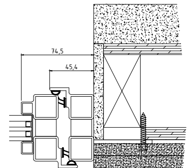
JAMB & STILE
