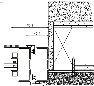
JAMB & STILE
